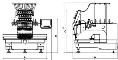
HCD3E-1501-40
