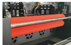
Rulli della calandra a caldo per il trasferimento della colla sul film B
